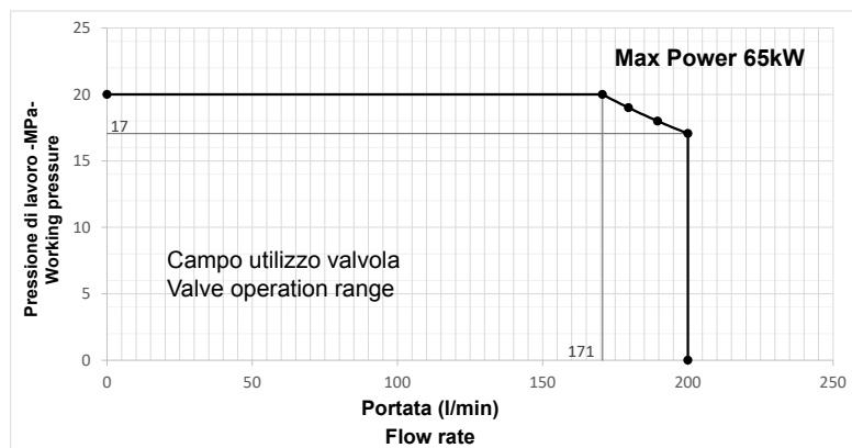
GRAFICO PRESSIONE IDAULICA / PORTATA - HYDRAULIC PRESSURE / FLOW RATE GRAPH GRAPHIQUE PRESSION HYDRAULIQUE / DÉBIT - HYDRAULIKDRUCK / DURCHFLOSSRATENDIAGRAMM
